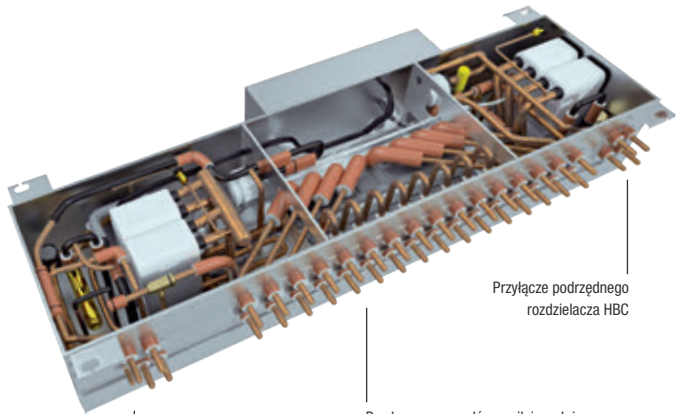
Przyłącza przewodów zasilających i powrotnych do systemu wodociągowego; dostępne są wersje z 8 lub 16 przyłączami.
